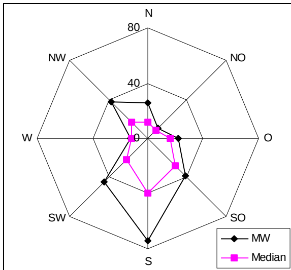
Abbildung 15: Mittelwert und Median der Herkunftsentfernung (km) der Wiederfunde aus Abbildung 14
